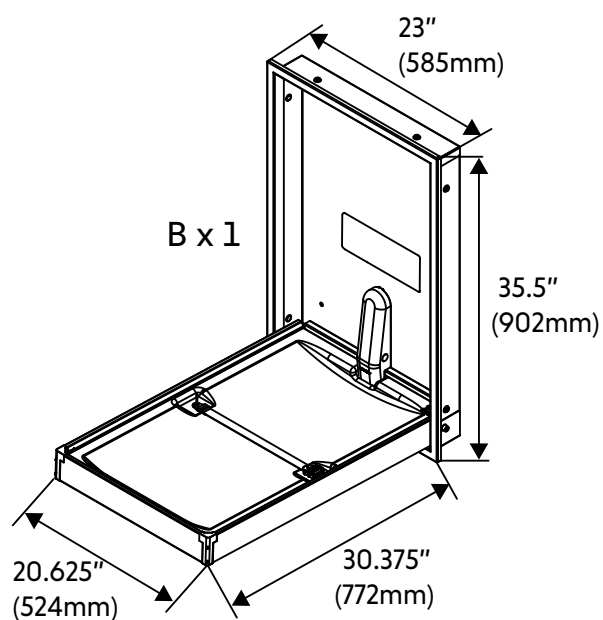
Montaje empotrado - Pagina 11
