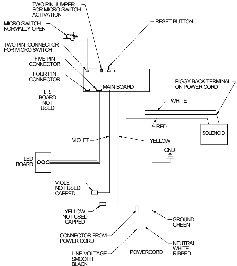
WIRING DIAGRAM 120 VOLT & 220 VOLT SINGLE & BI-LEVEL MICRO SWITCH ACTIVATION
