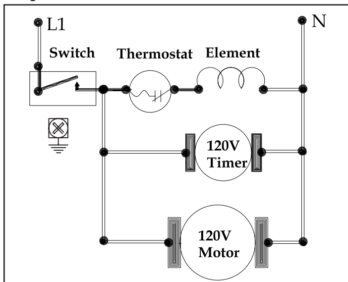
Diagrama de Cableado - Modelo RA5
