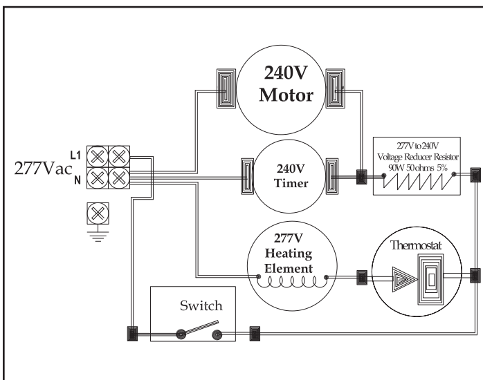
Schéma de câblage - Modèle RA57
