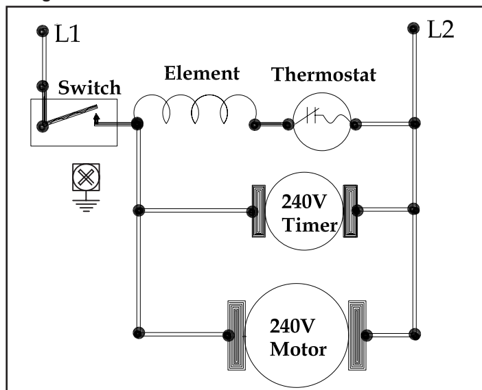
Diagrama de Cableado - Modelo RA54/RA548
