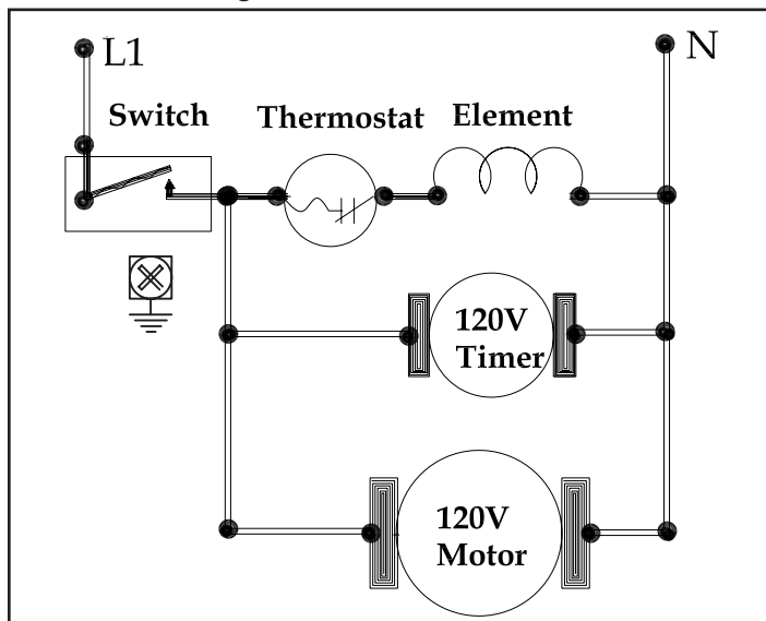
Schéma de câblage - Modèle RA5
