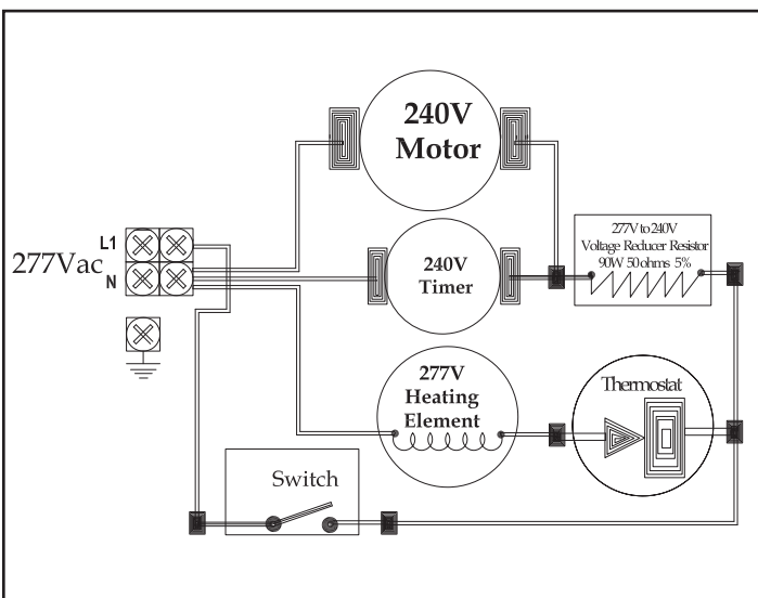
Diagrama de Cableado - Modelo RA57
