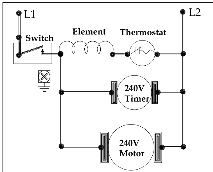
Schéma de câblage - Modèle RA54/RA548
