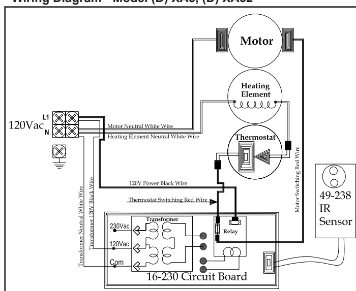
Wiring Diagram - Model (D) XA5, (D) XA52
