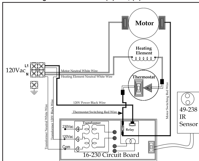
Verdrahtungsschema - Modell (D)XA5, (D)XA52
