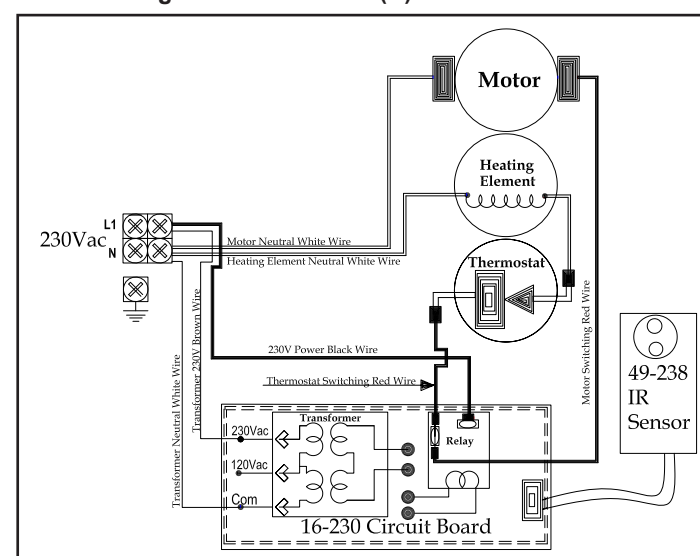
Verdrahtungsschema - Modell (D)XA57
