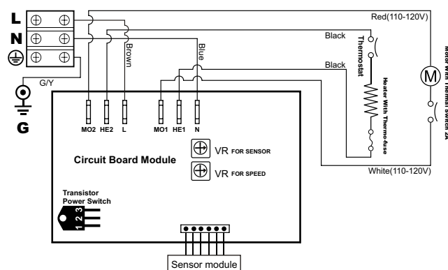
208~240V
